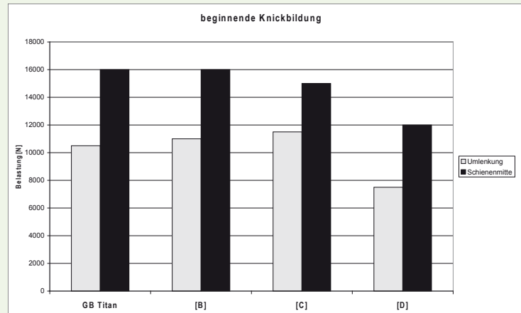
Abb. 3: beginnende Knickbildungen
