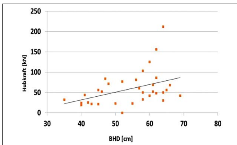
Diagramm 2: Verhältnis der Hubkraft zum BHD für Buchen im Winter
