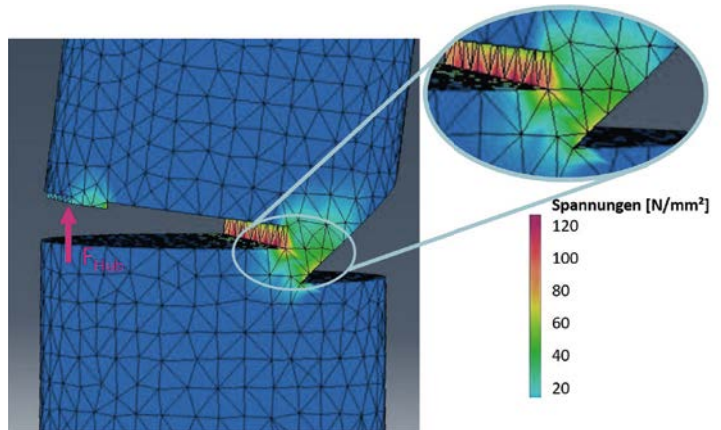
Abbildung 5: Simulation der Spannungen beim Fällen in der Bruchleiste
