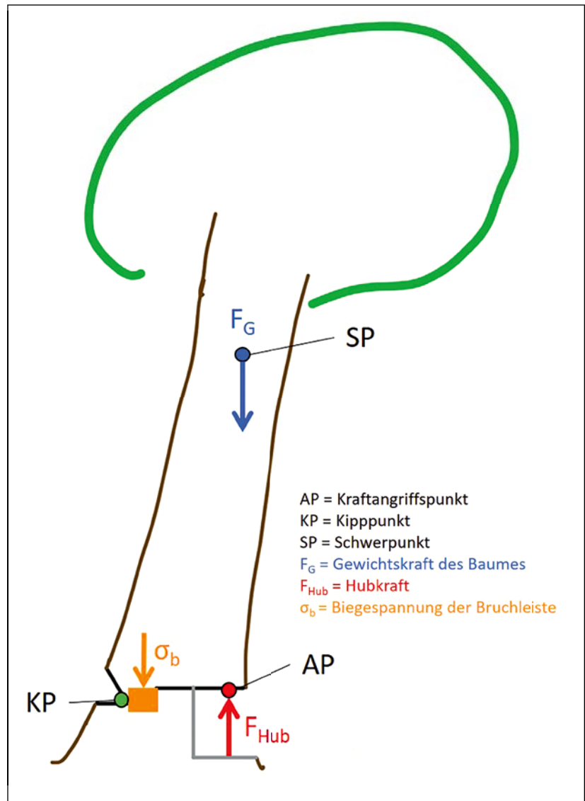
Abbildung 1: Freischnitt der dominierenden Kräfte bei der Baumfällung (unter Verwendung technischer Fällhilfen)
