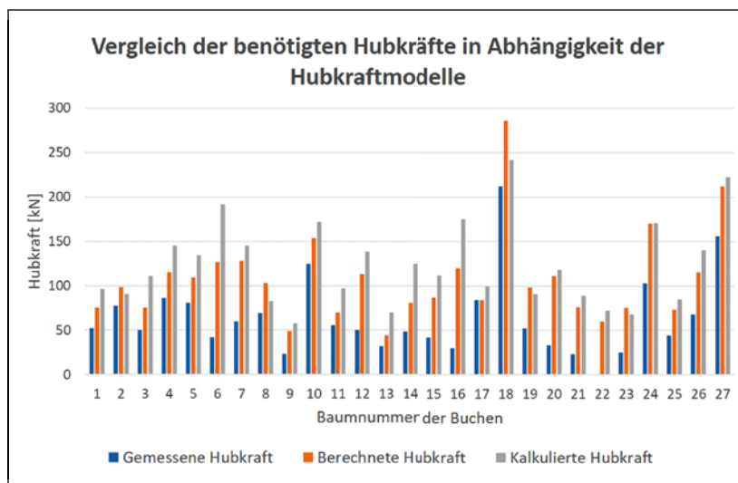
Diagramm 1: Vergleich der ermittelten Hubkräfte
