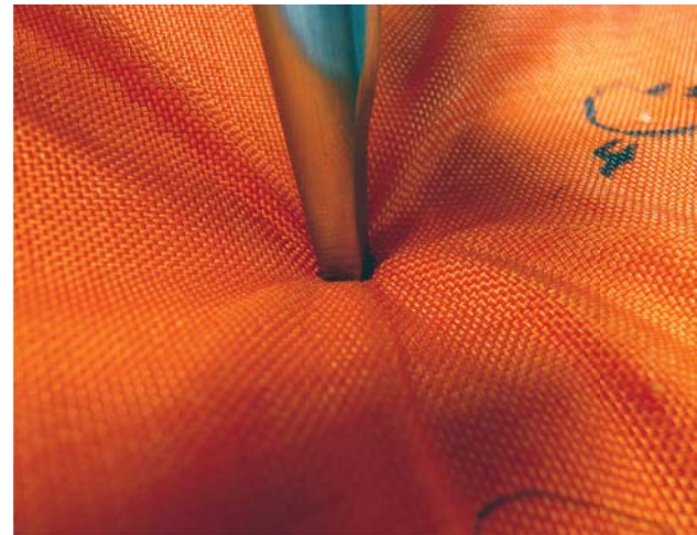
Abbildung 4: Dieses Hosengewebe wurde deutlich sichtbar durchschlagen und hat damit das Testziel nicht erreicht.
