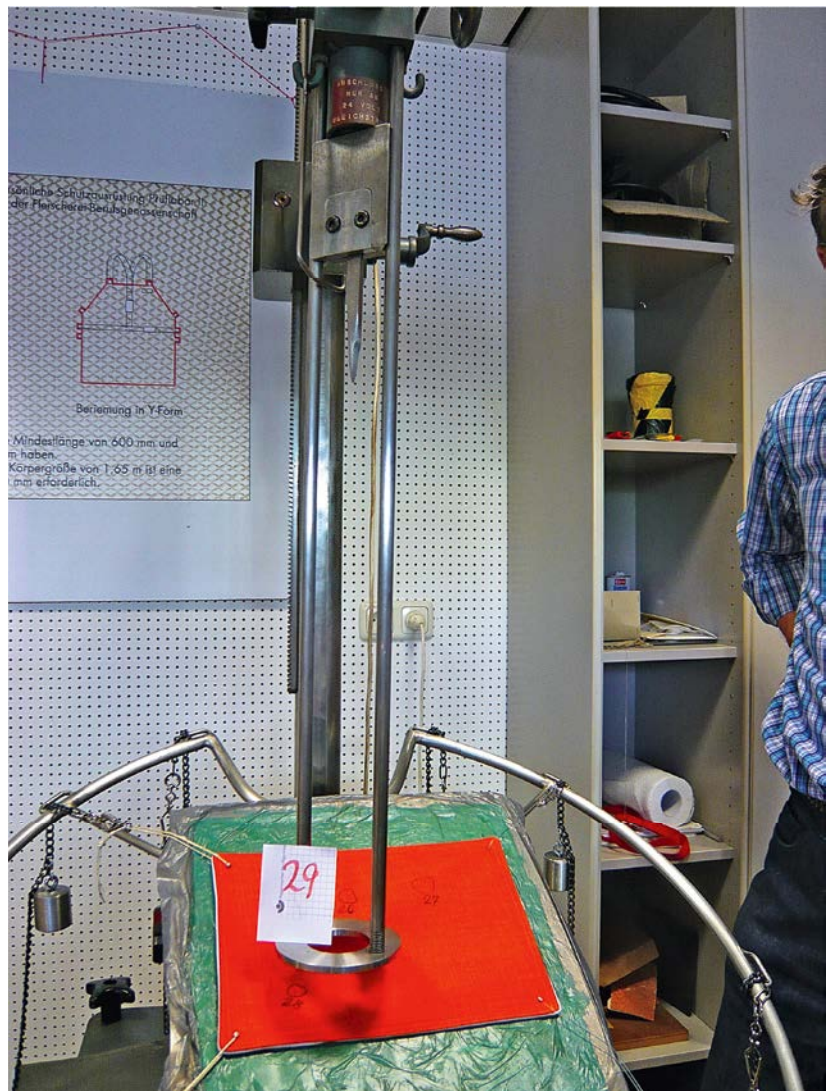
Abbildung 2: Der gewichtsbelastete Prüfzahn fällt nach Abschalten eines Elektromagneten auf das in schrägem Winkel aufgespannte Prüfmuster. Dadurch wird der Tatsache Rechnung getragen, dass Angreifende Keiler in einer halbkreisförmigen Bewegung schlagen.
