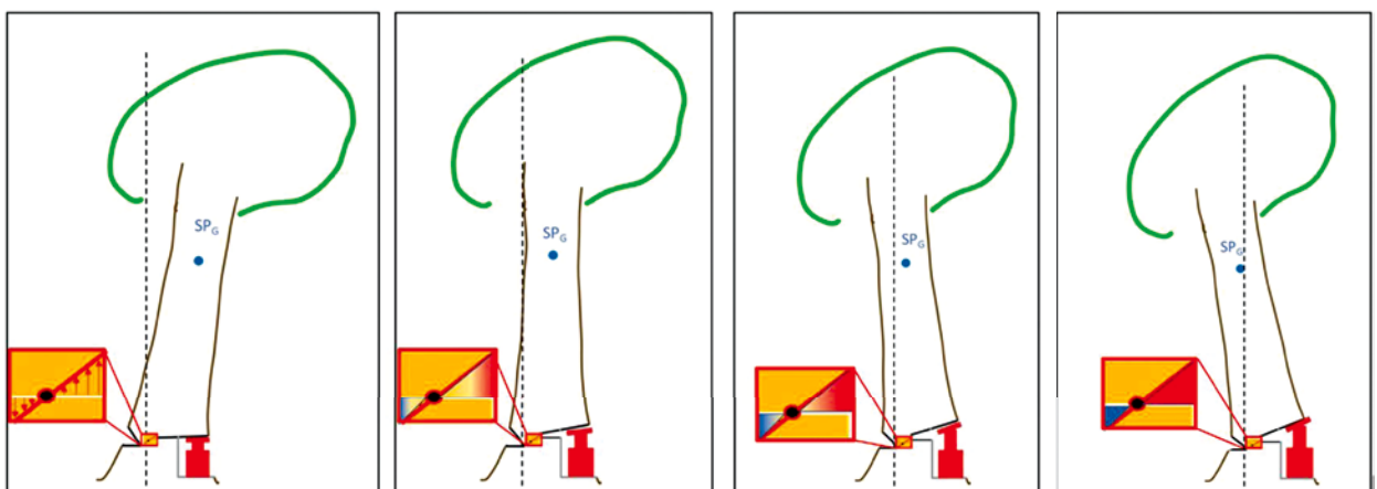
Abbildung 6: Schema der Spannungen in der Bruchleiste bei unterschiedlichen Hubhöhen der Fällhilfe
