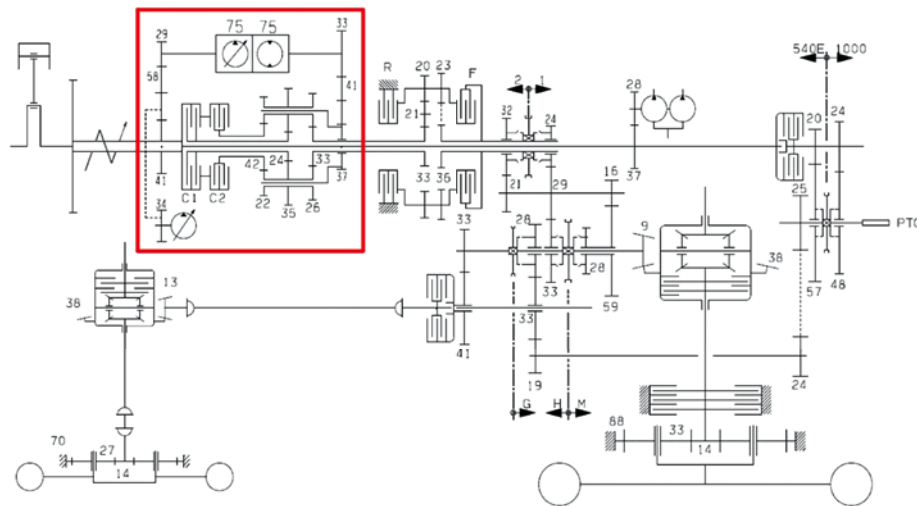
Abbildung 5: Schemazeichnung des Stufenlosgetriebes Bauart Valtra; rot gekennzeichnet die Leistungsverzweigungsbaugruppe. Untenliegend sind 2 Planetengetriebestufen angeordnet und darüber ist die hydrostatische Wandler-einheit zur stufenlosen Drehmoment-wandlung dargestellt (Bild Valtra).
