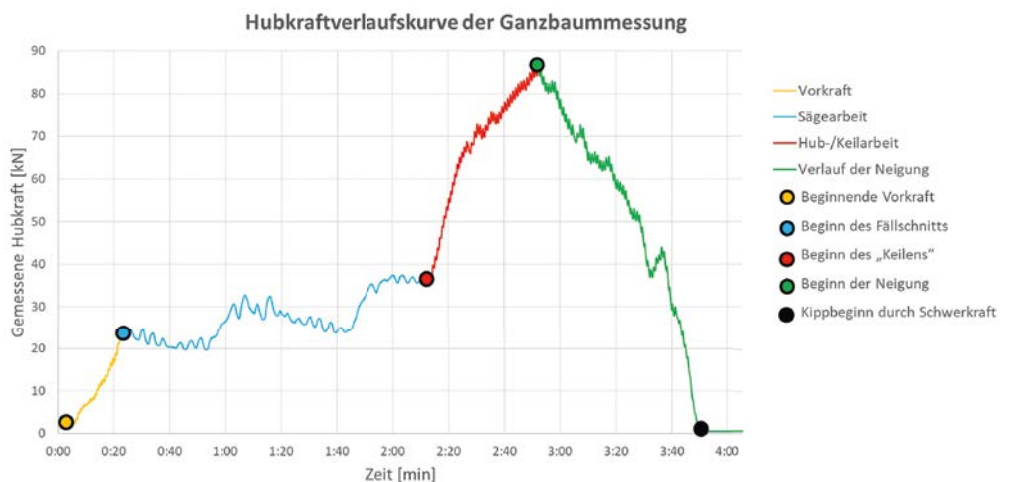
Abbildung 12: Kraftverlauf bei der Fällung
