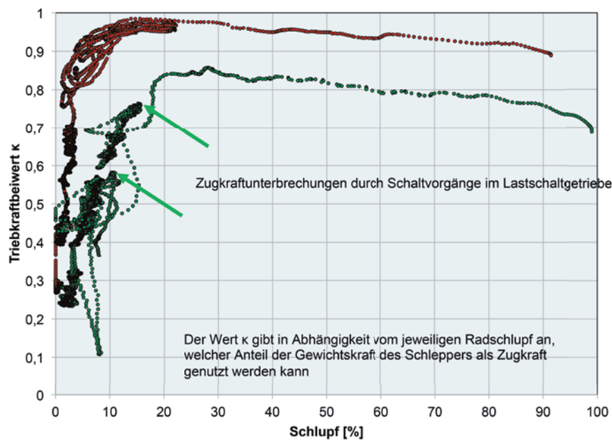
Abbildung 6: Vergleich des Triebkraftbeiwerts \kappa der Maschine Valtra N 174 Active (grün) mit dem ermittelten Triebkraftbeiwert \kappa der Maschine Valtra N 174 Direct (rot) (Messungen während der KWF-Gebrauchswertprüfung).
