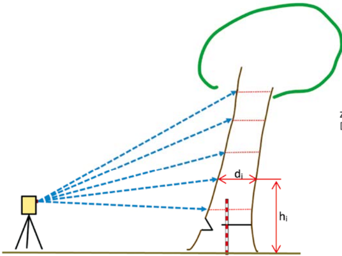
Abbildung 7: Schema der Lasermessung der Geometrie des Stammes.
